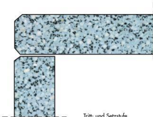
Tritt- und Setzstufe (rechtwinklig) mit Nut 4/4cm stark
