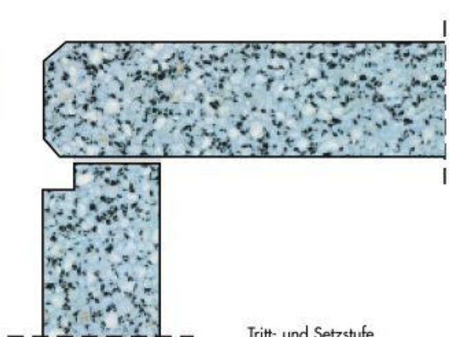
Tritt- und Setzstufe (rechtwinklig) mit Falz 4/4cm stark
